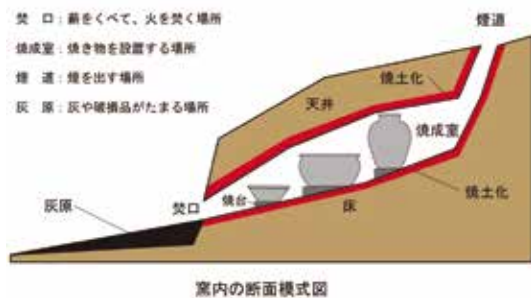
窯内の断面模式図
